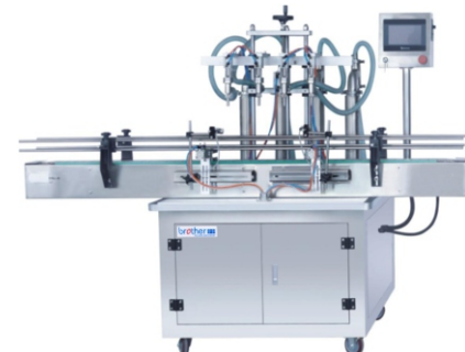
AYF/4D(4 Nozzle) Automatic Liquid Filling Machine 自动液体灌装机 Filling Capacity/灌装容量: 10-100ml or 30-300ml or 50-500ml or 100-1000ml or 250-2500ml or 500-5000ml Capacity/工作效率: 30-60bottle/min.
